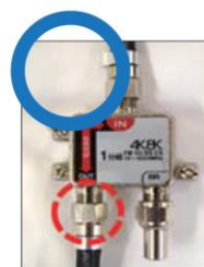
シールド性能の高い接続例
